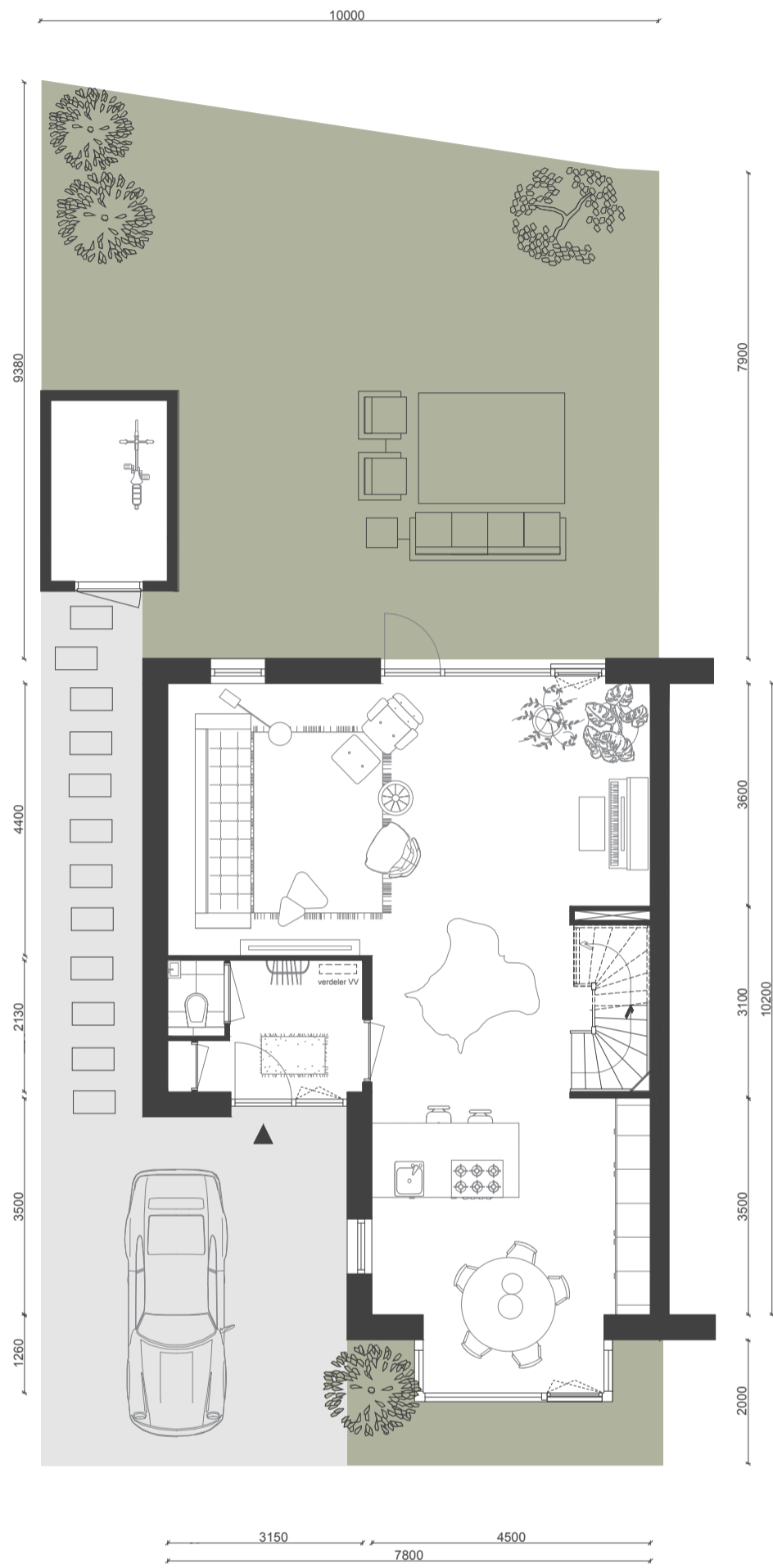
begane grond
