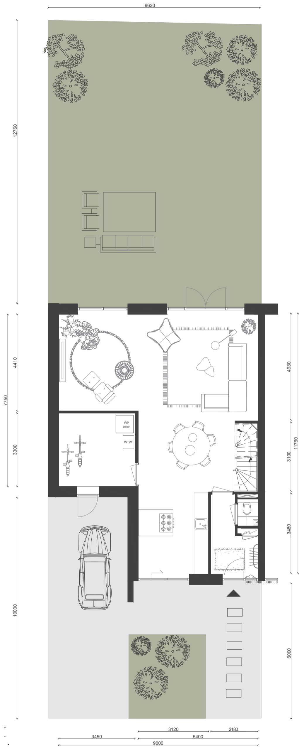
begane grond SCHAAL 1:100
