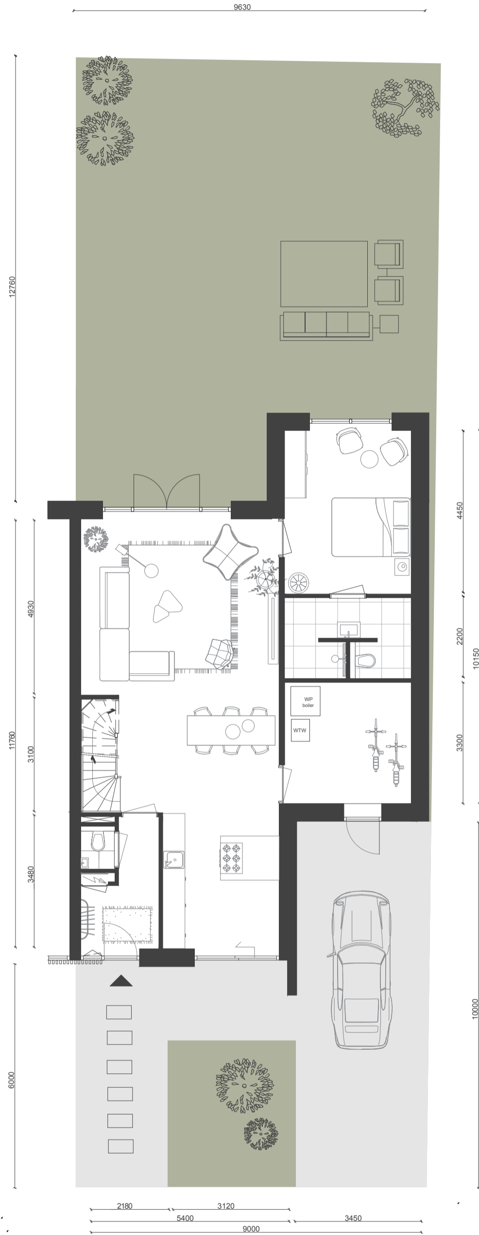
begane grond SCHAAL 1:100
