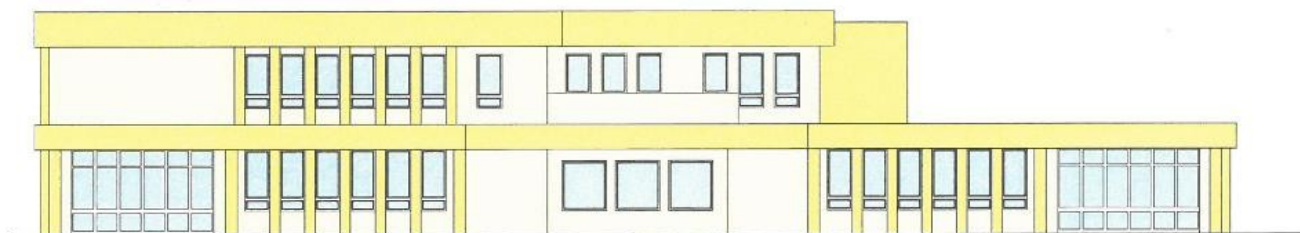
POHLED JIŽNÍ
