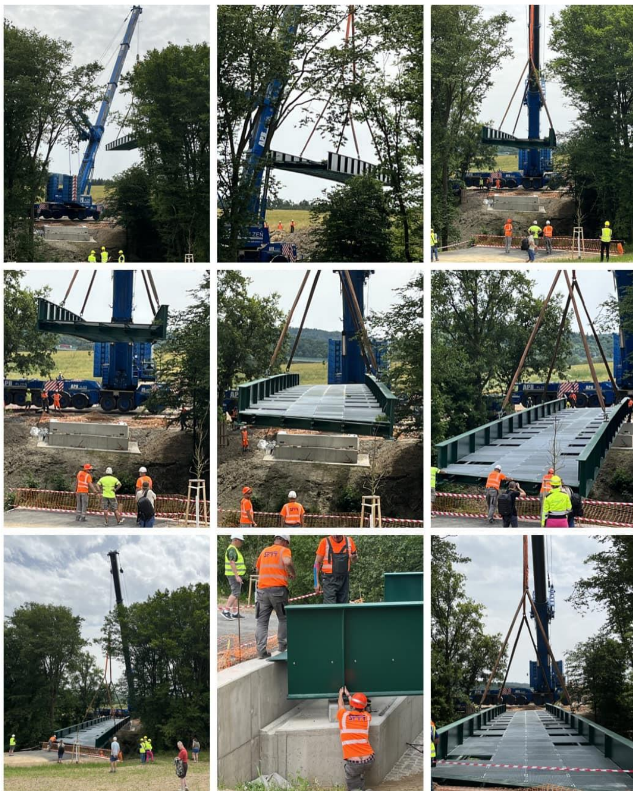
Usazování lávky přes rokli v lokalitě V Lahošti. 20. června 2024.
