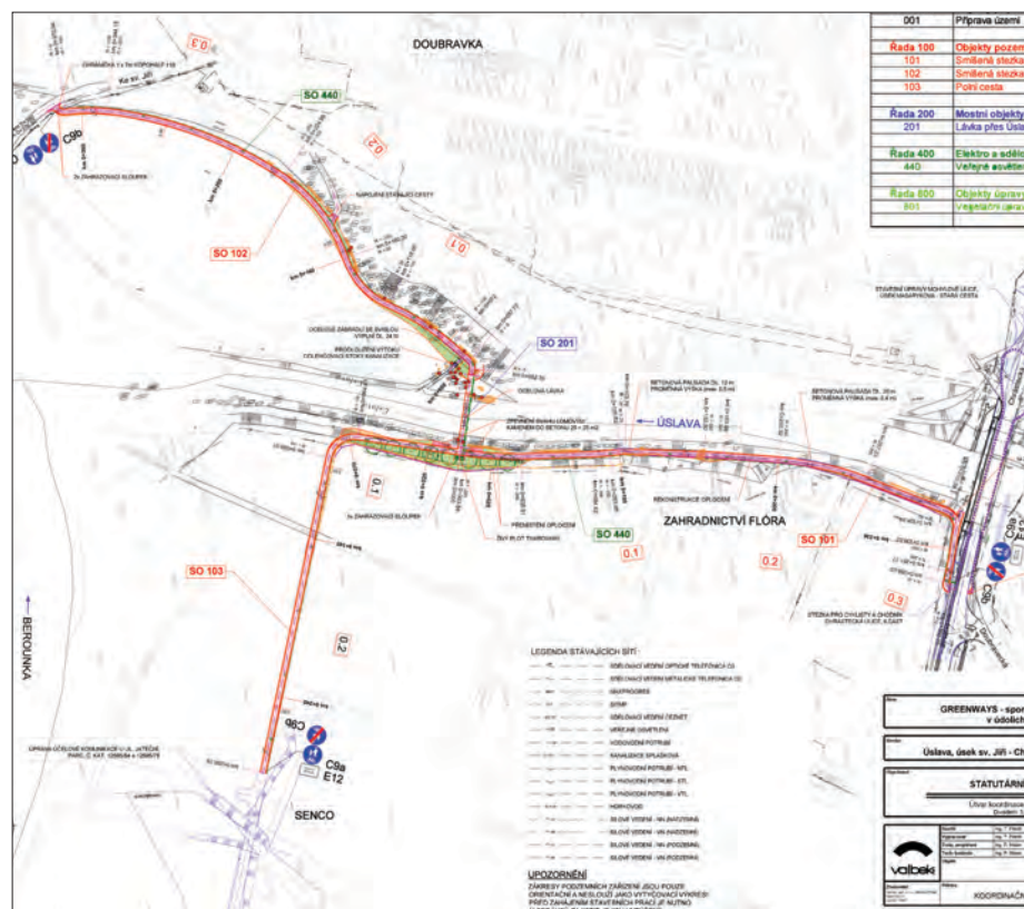
Situace budoucího napojení prvního úseku s nově vybudovanou lávkou.
