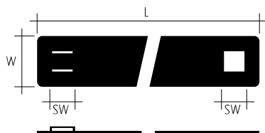
MOCOWANIE POJEDYNCZE
