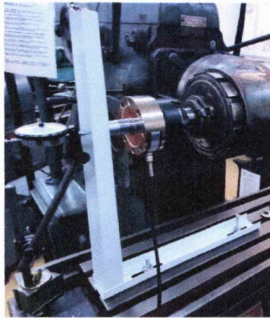
Слика 2. Изглед испитног места
