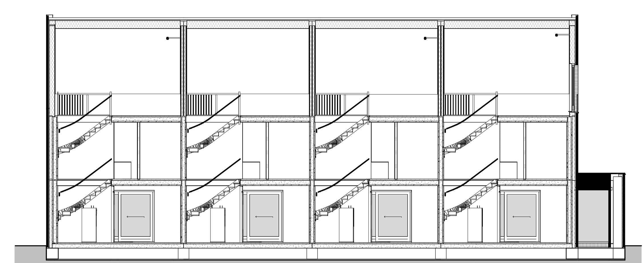
doorsnede B-B 1:100
