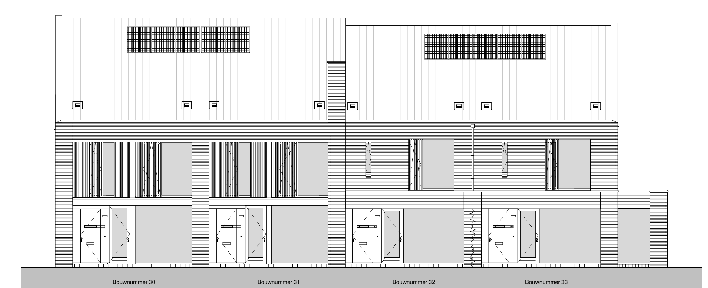
voorgevel 1:100
