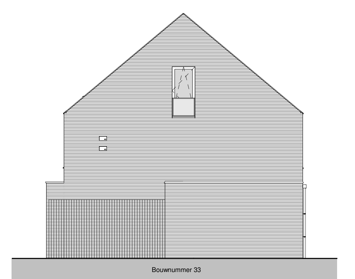
rechtgevel 1:100
