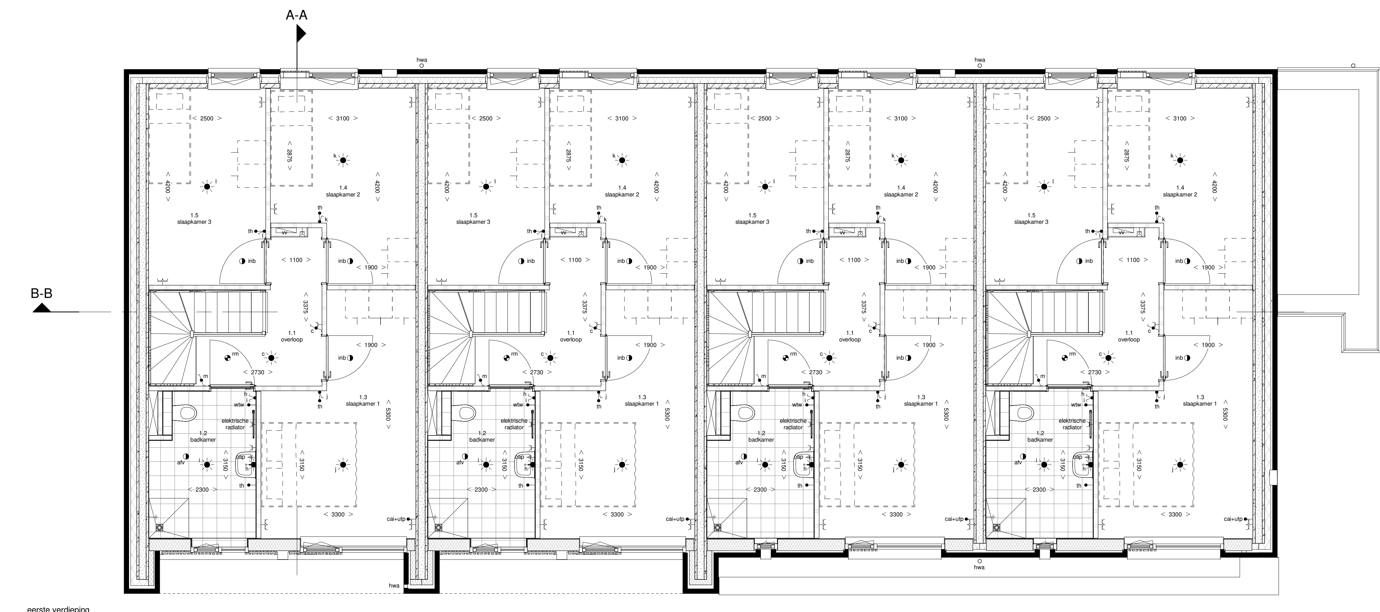
eerste verdieping 1:50
