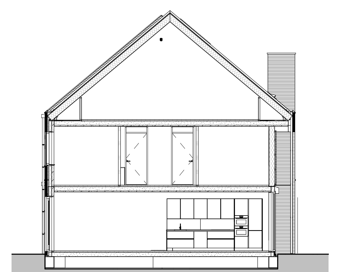
doorsnede A-A 1:100
