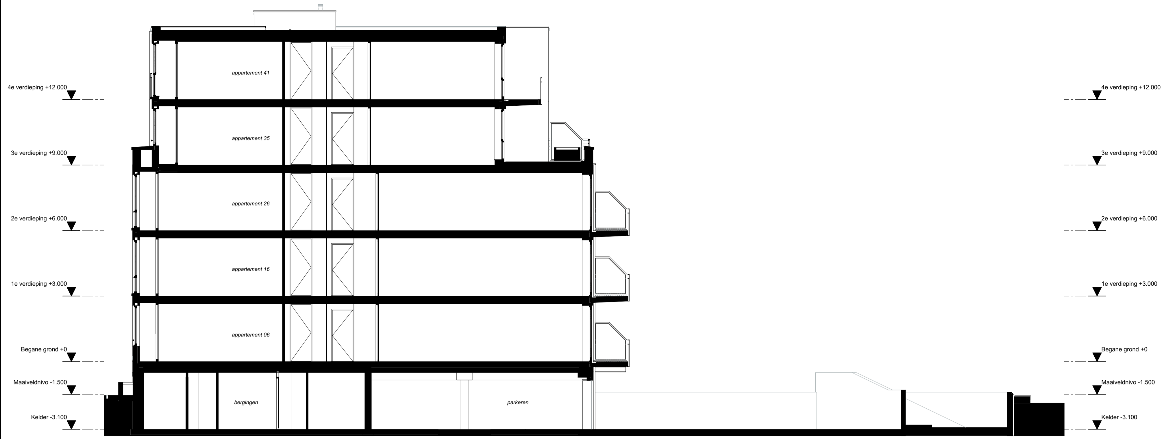
Doorsnede A1
