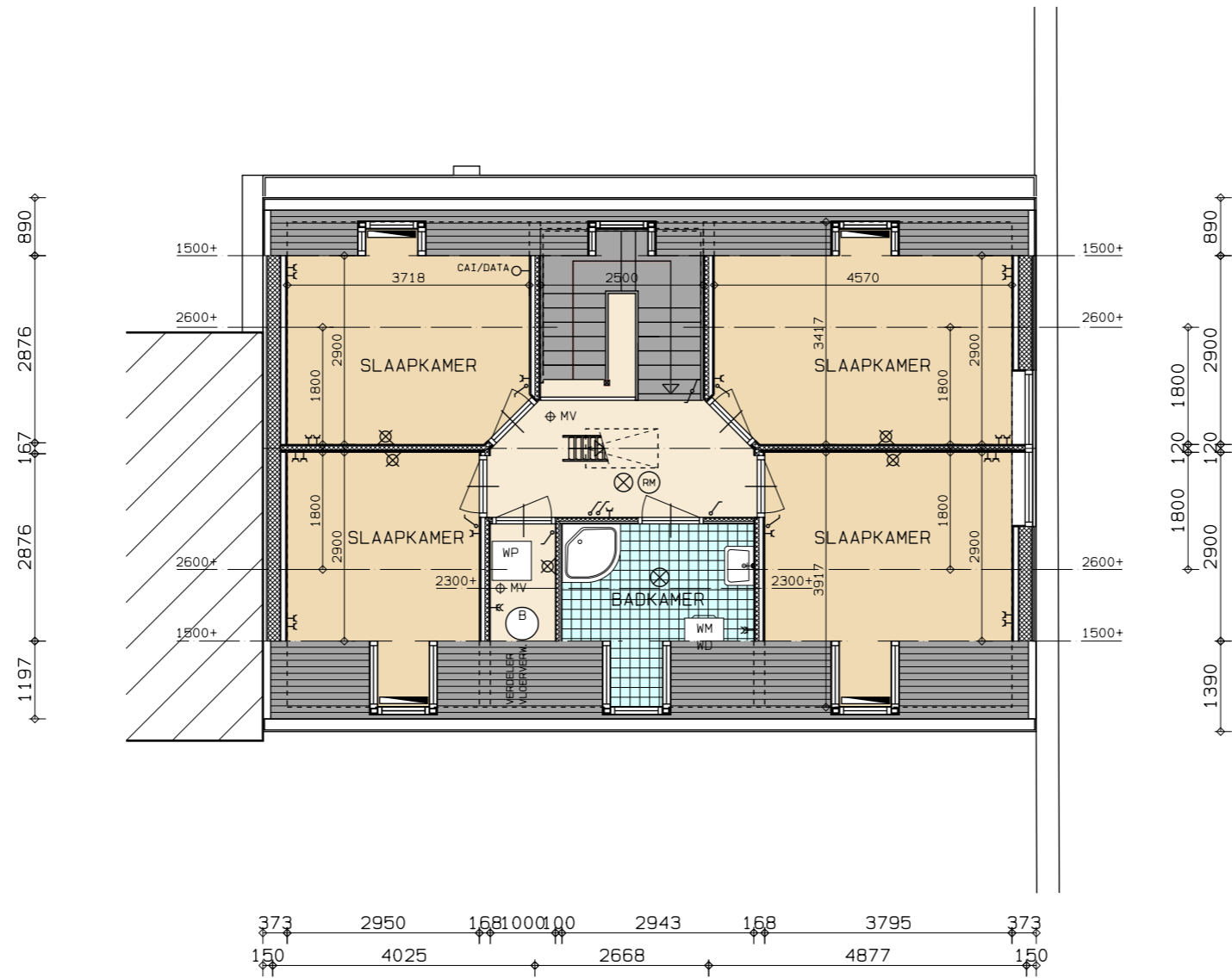
VERDIEPING > BOUWNR. 3 (TYPE: D) OPTIE 2 SLAAPKAMERS
