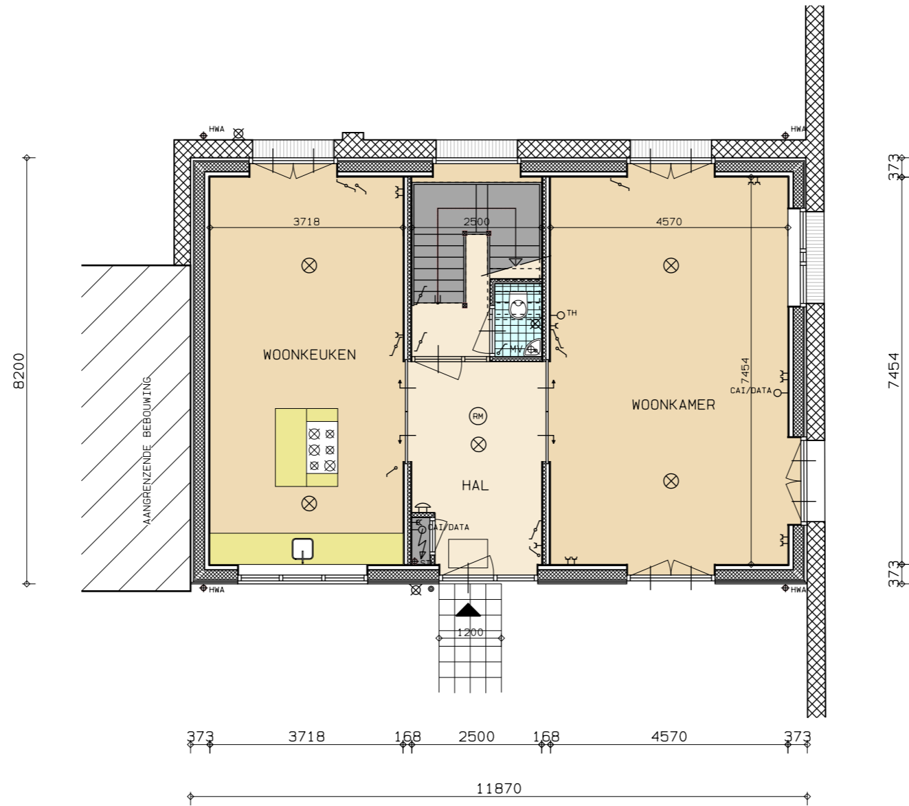
BEGANE GROND > BOUWNR. 3 (TYPE: D) VARIANT KEUKEN
