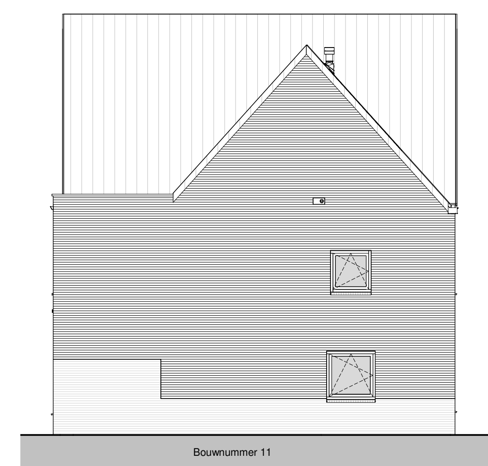
rechtergeve 1 : 100
