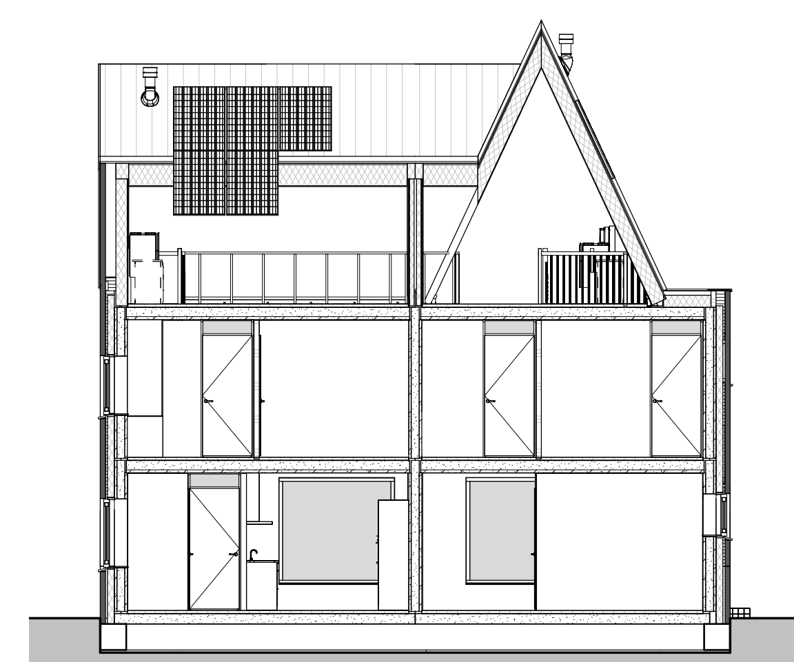
doorsnede E 1 : 100
