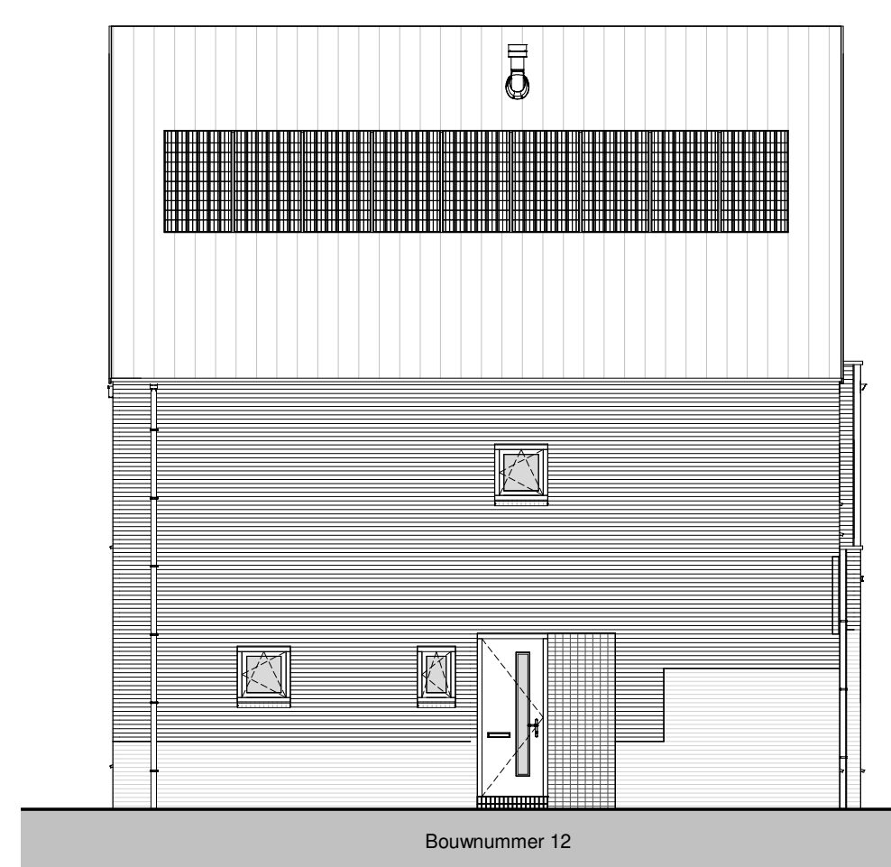
linkergeve 1 : 100
