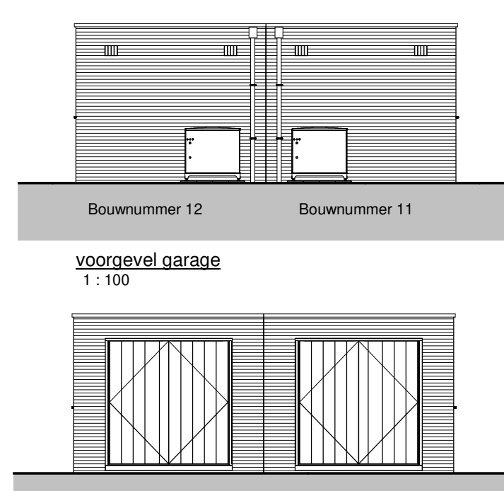
achtergevel garage
