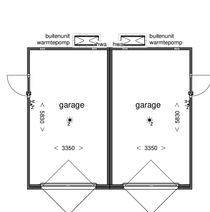
platted 1 : 100
