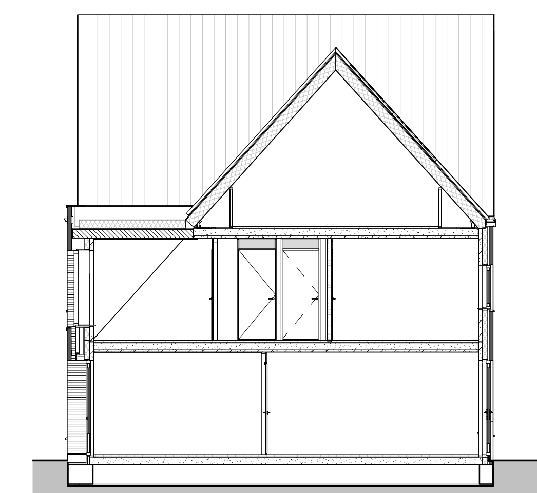
doorsnede E 1 : 100
