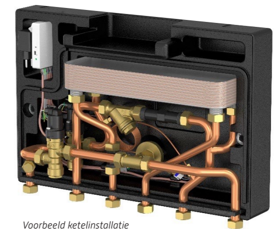
Voorbeeld ketelinstallatie en warmte afgifteset
