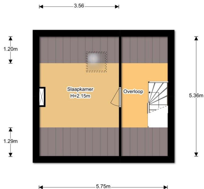
2e Verdieping
