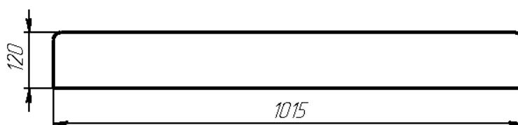
Рисунок 7.4. Креслення фільтруючого елемента
