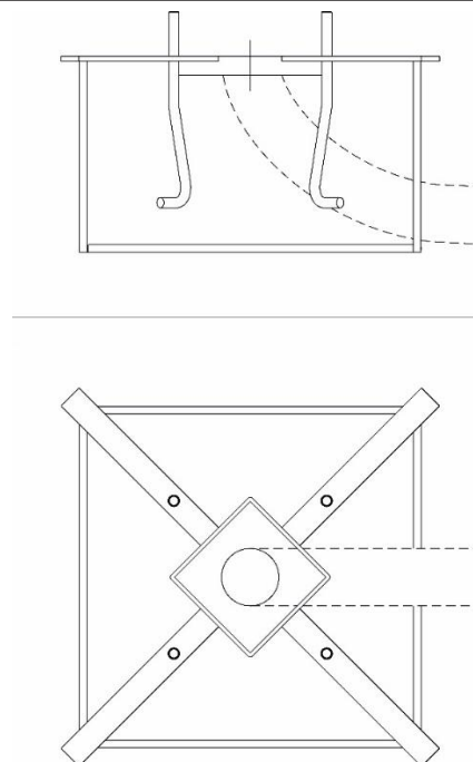
Рисунок 5.4. Фундамент станції
