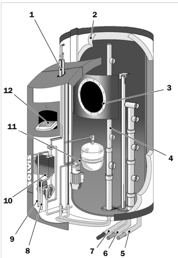
Abb. 4: Pufferspeicher SolvisMax Futur LF
