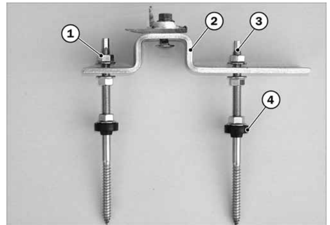
Fig. 51 : fixation sur toiture ADH-W
