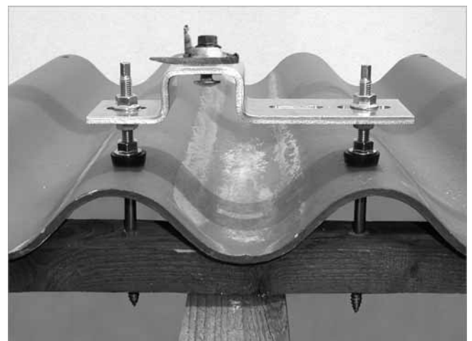
Fig. 60 : fixation sur toiture vissée (méthode C)
