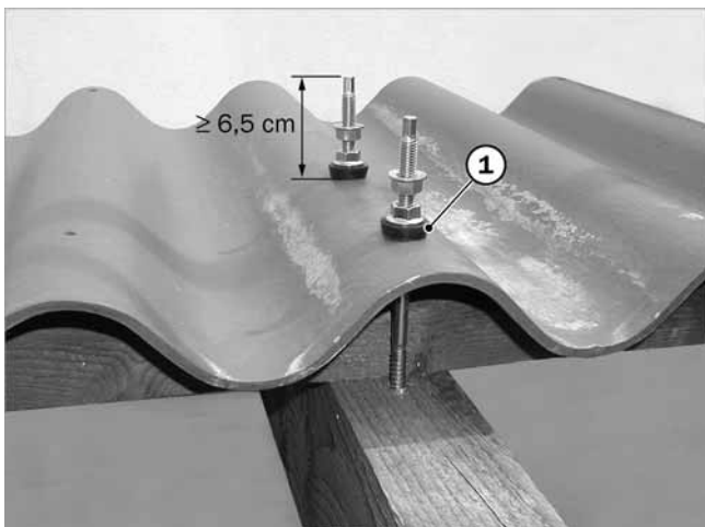
Fig. 33: Ambos tirafondos en el cable (método A)
