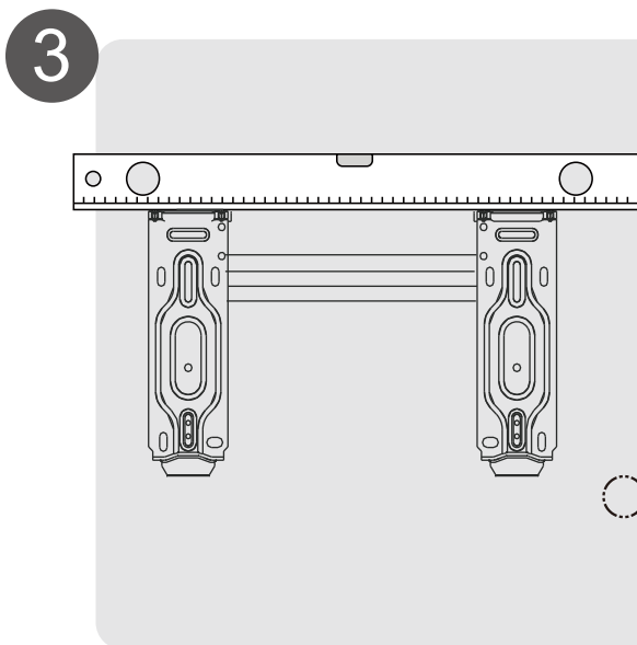
Fije la placa de montaje
