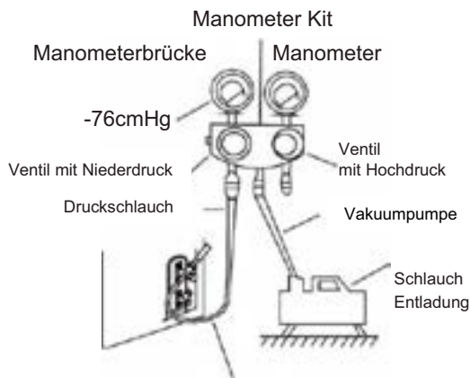
Niederdruckschlauch
