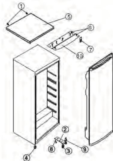
FIGURA 1 – REPRESENTA LA POSICIÓN DE LOS COMPONENTES ANTES DEL CAMBIO DE LA PUERTA.
