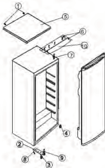
FIGURA 1 – REPRESENTA LA POSICIÓN DE LOS COMPONENTES ANTES DEL CAMBIO DE LA PUERTA.
