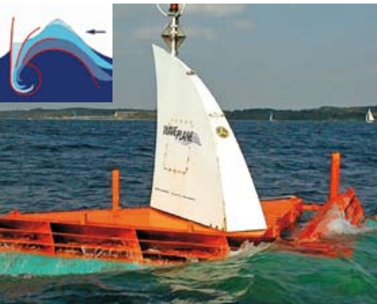
BølgeHøveln i Mariager Fjord i 1999, hvor den blev brugt til at pumpe iltet vand ned til den døde bund. Tegningen øverst viser, at de vandrette lameller skærer bølgen i skiver og presser hastigheden op og ind i et vandret rør. Bølgehøveln klarede vinterstormen 1999
