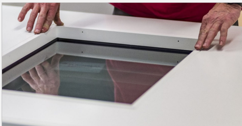
Montaggio del vetro con listelli fermavetro all'interno
