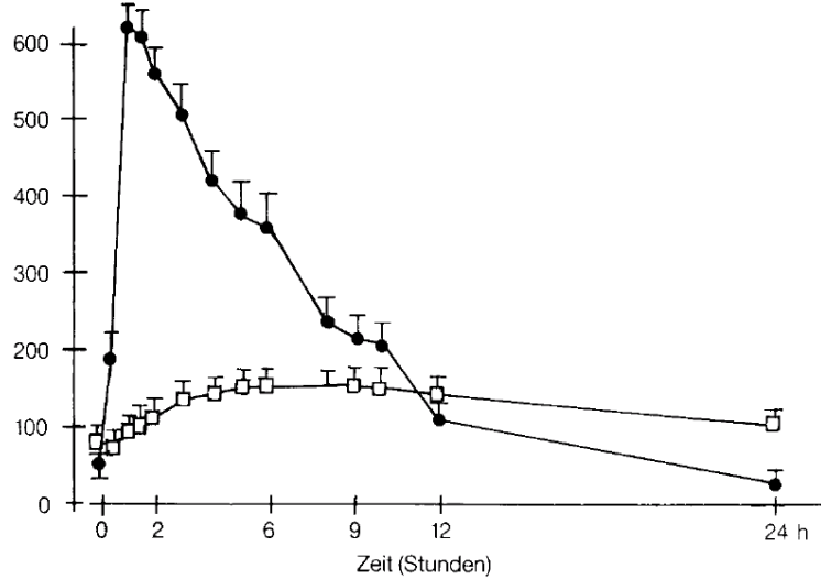
Plasmakonzentration von Metoprolol (nmol/l)
