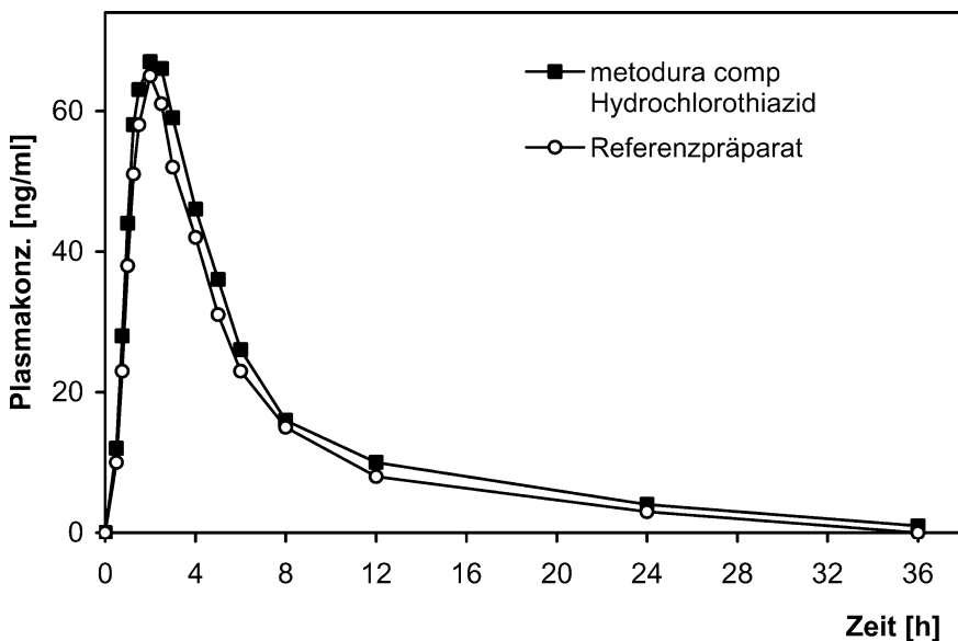
Abbildung 2: Mittlere Plasm Spiegelverläufe im Vergleich zu einem Referenzpräparat in einem Konzentrations-Zeit-Diagramm:
