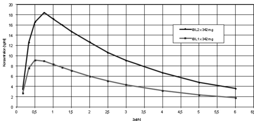
Verlauf der Plasmakonzentrations-/Zeitkurve von S-Ibuprofen (wirksames Enantiomer von Ibuprofen) nach Gabe von 342 mg bzw. 684 mg Ibuprofen, DL-Lysinsalz (1 bzw. 2 Filmtabletten)
