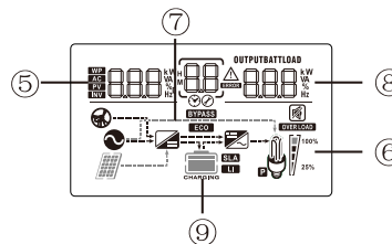
LCD display
