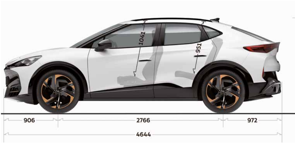
AFMETINGEN
