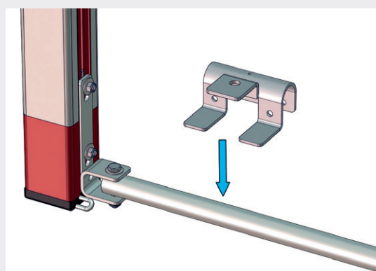
Focus fixation patte d'ancrage sur arceau
