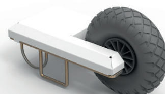
Roue gonflable et système de fixation
