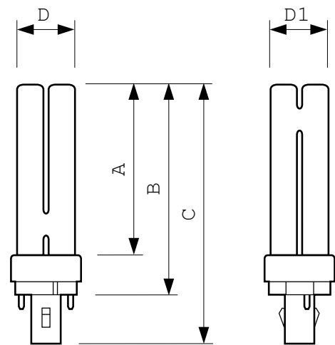
G24d-1/G24d-2/G24d-3, 2P
