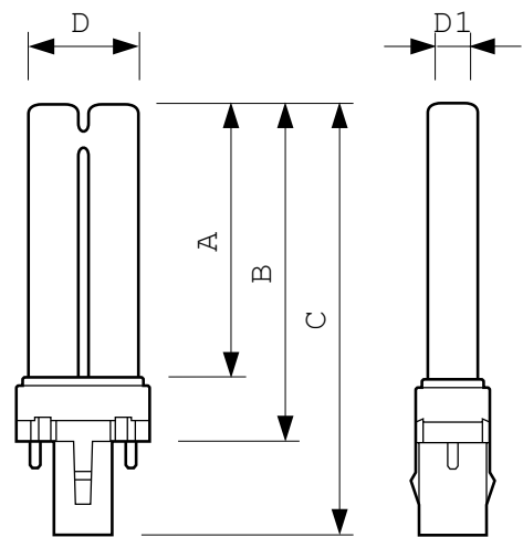
G23/GX23, 2P
