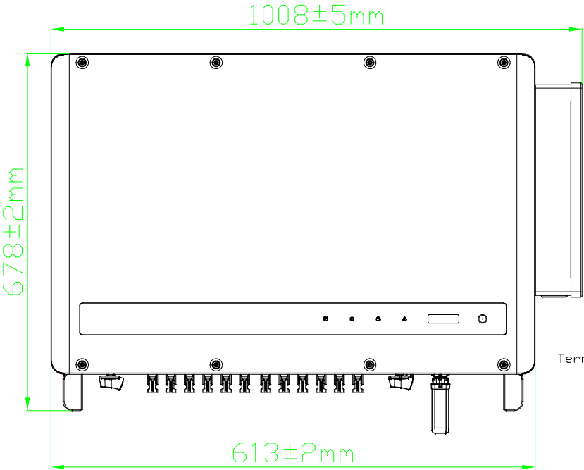
Vista frontale
