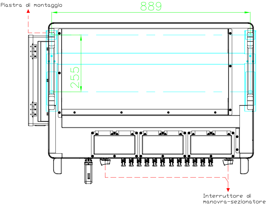
Vista posteriore
