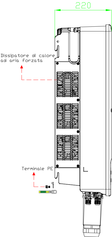
Vista laterale
