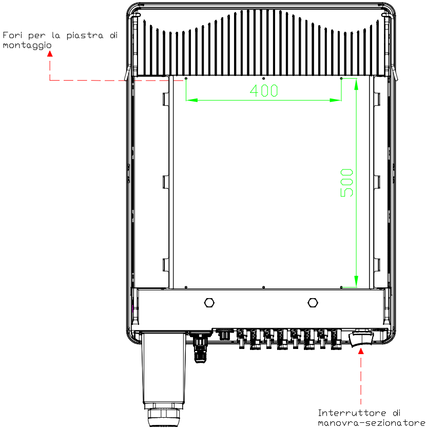
Vista posteriore
