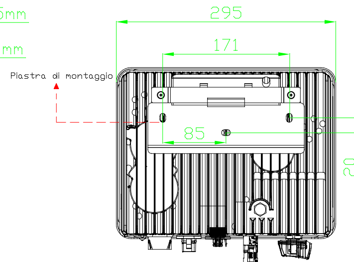
Vista posteriore
