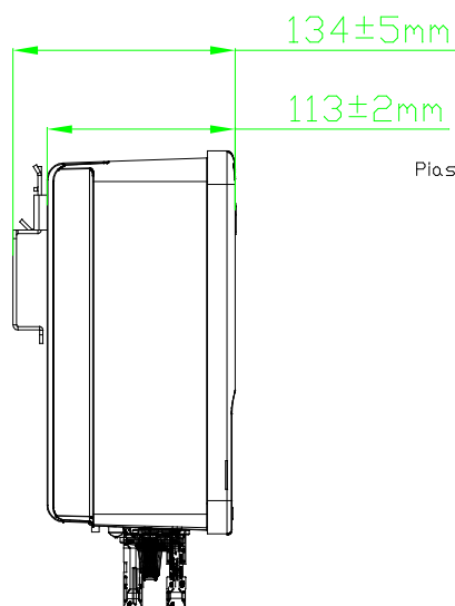
Vista laterale
