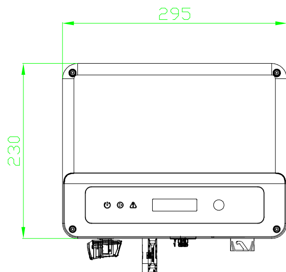
Vista frontale
