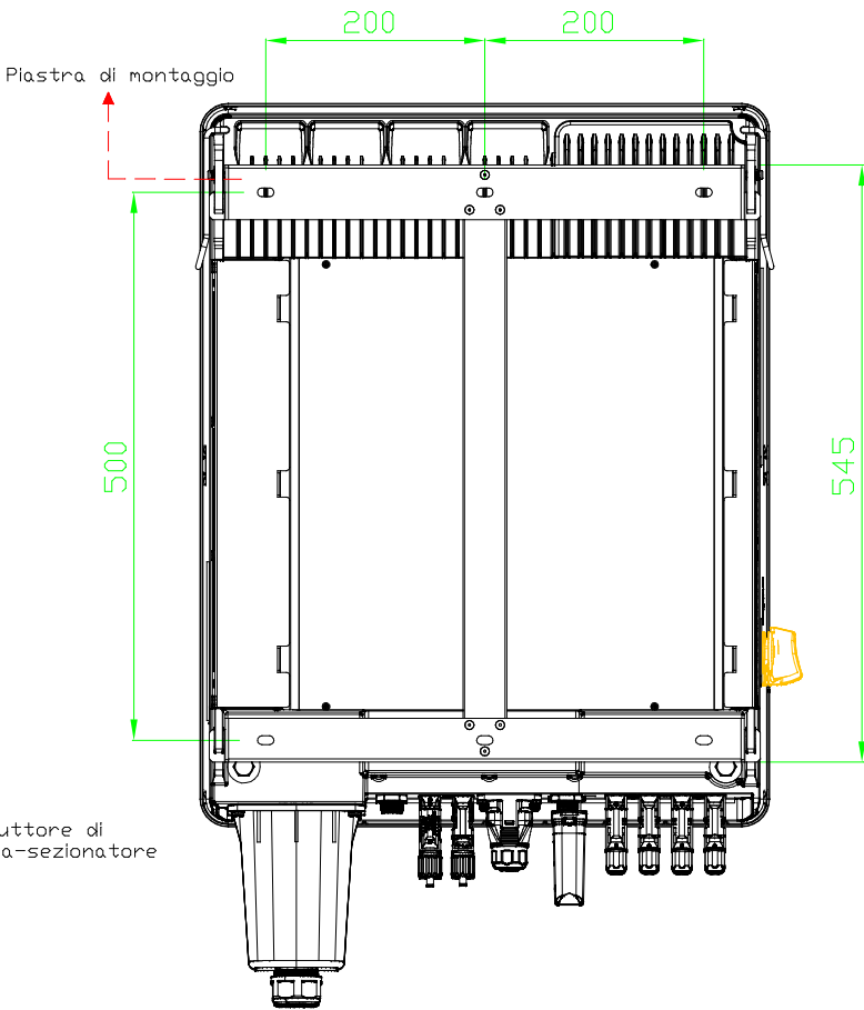
Vista posteriore
