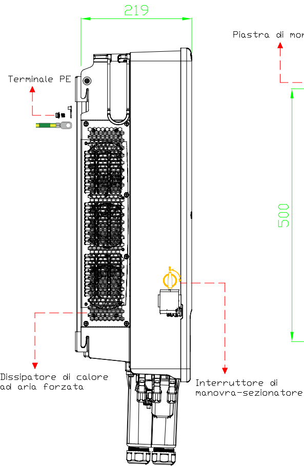
Vista laterale
