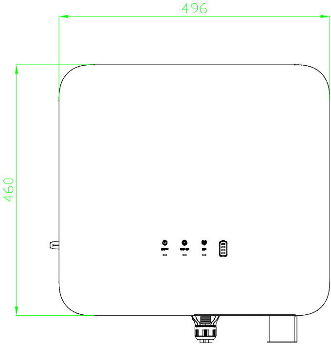
Vista frontale
