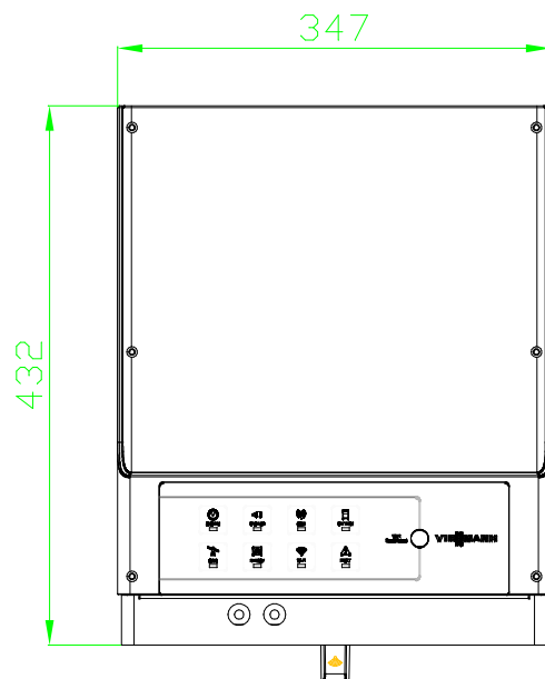
Vista frontale
