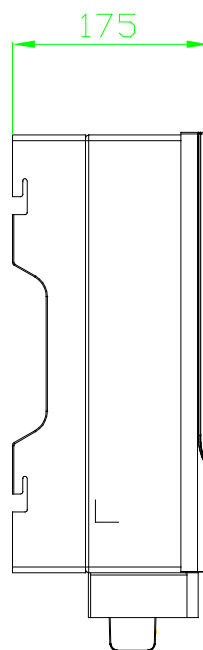
Vista laterale
