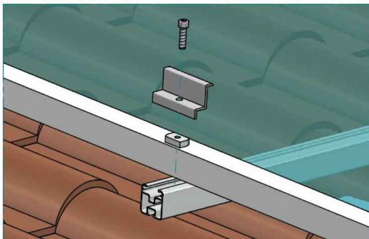
Morsetto fermapannello FINALE con blocchetto eccentrico - AL 6060 T6
