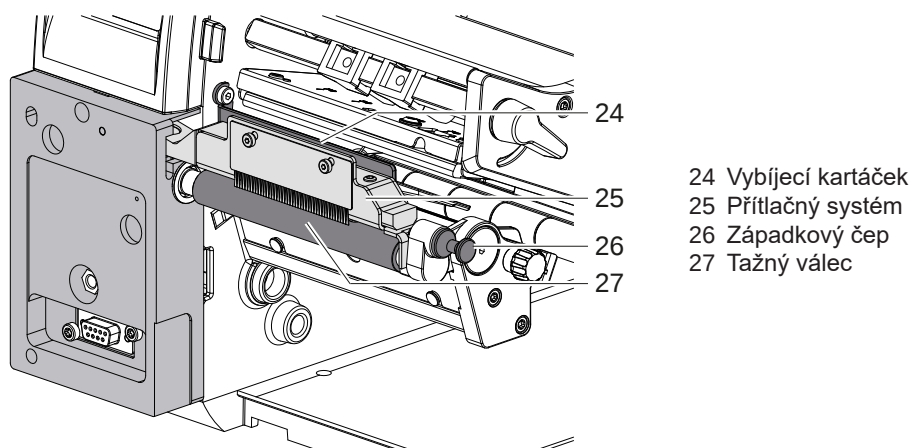
Obrázek 6 Separátor na SQUIX MT
