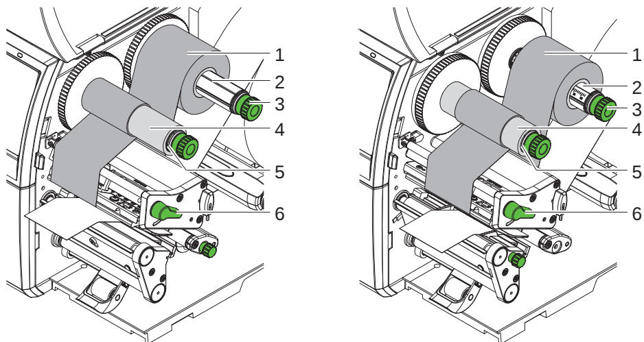
Obrázek 25 Vložení barvicí pásky
