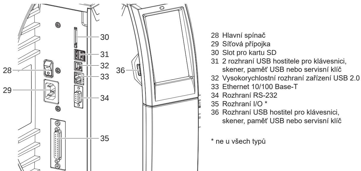
Obrázek 7 Přípojky
