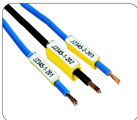
PFC och PTZ+ hållare som ledningsmärkning.
