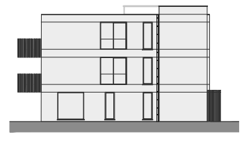
BLOK B - ZIJGEVEL LINKS
