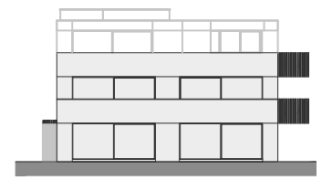
BLOK B - ZIJGEVEL RECHTS
