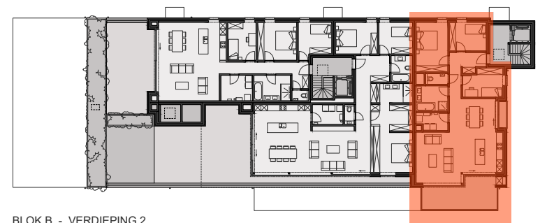
BLOK B - VERDIEPING 2
