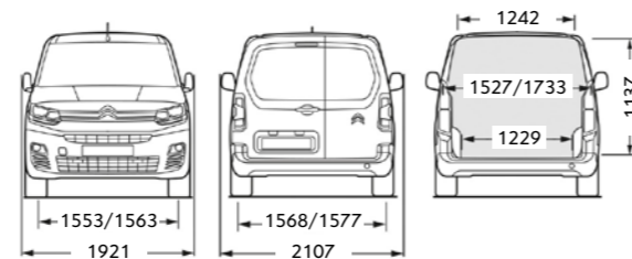
Afmetingen in millimeters.
