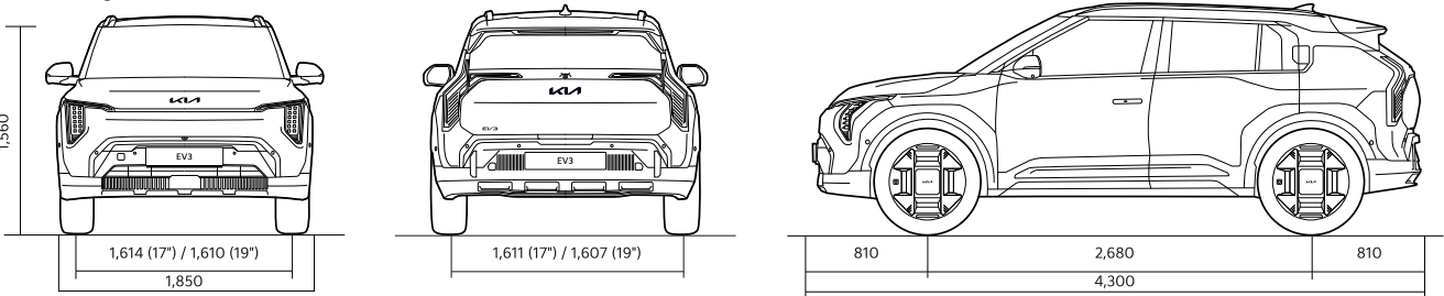
Afmetingen GT-Line
