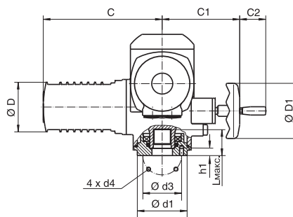
Исполнение N без центровки
