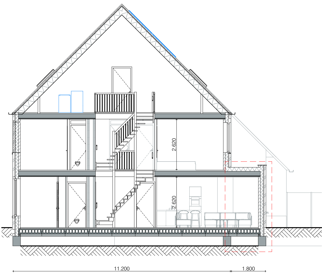
Doorsnede
