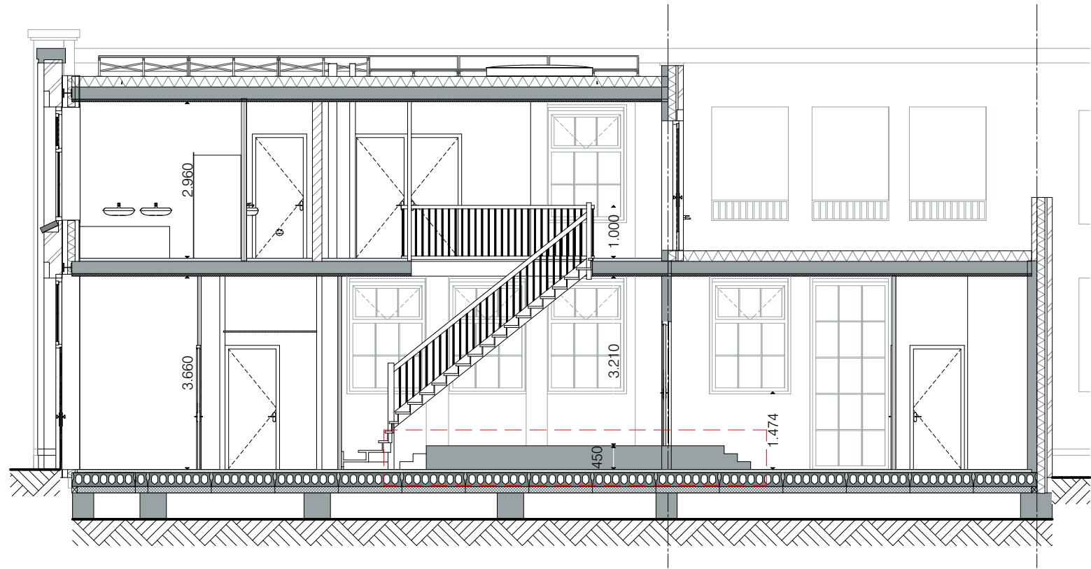
Doorsnede
