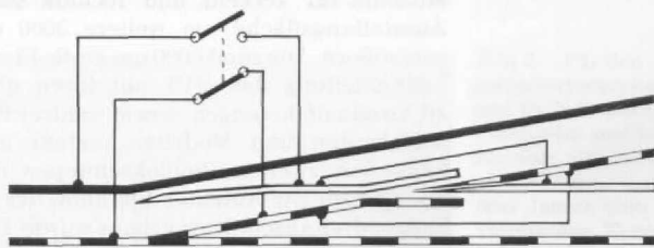
Bild 2. Umbau nach Christian Schäffer: Stoppweiche.
