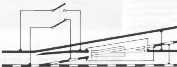
Bild 1. Minitrix-Weiche in Originalausführung: Durchfahrtsweiche.
