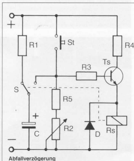
Bild 2. Abfallverzögerung (links) und Anzugverzögerung (rechts).
