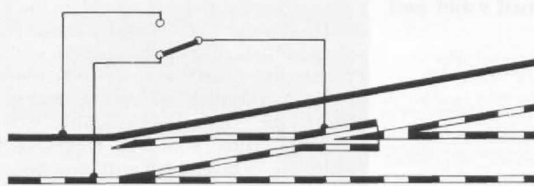
Bild 3. Alternative Herzstückpolarisierung einer Stoppweiche.
