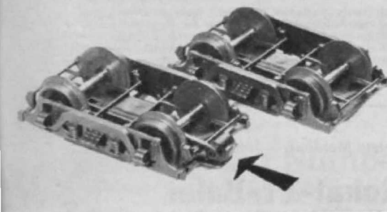
► Abb. 4. Das Drehgestell mit normaler (links) und verkürzter Kupplung (rechts). Die Noppen an der Kupplungsdechsel an den mit einem Pfeil gekennzeichneten Stellen mit den Fingernägeln o. ä. zusammendrücken und Kupplung bis zum Einrasten einschieben. Beim Herausziehen genügt ein kurzer Ruck.
